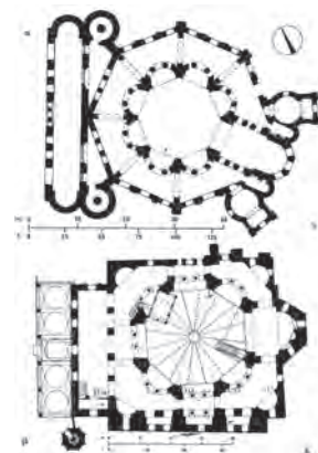
2. Κάτοψη περίκεντρου ναού α) Αγ. Βιταλίου, Ραβέννα. β) Αγ. Σεργίου και Βάχχου, Κωνσταντινούπολη.
