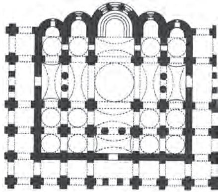
Κάτοψη ναού Αγ. Σοφίας Κιέβου, ρυθμός σταυροειδής με θόλο.
